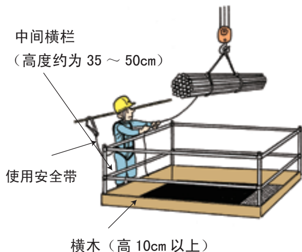
开口部位附近的作业
