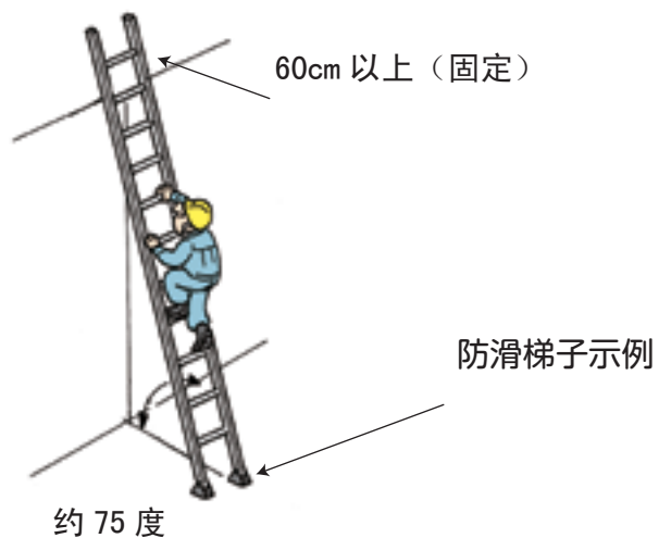
使用梯子的作业
